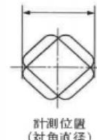
<ちくとうの最小直径値の計測方法>
